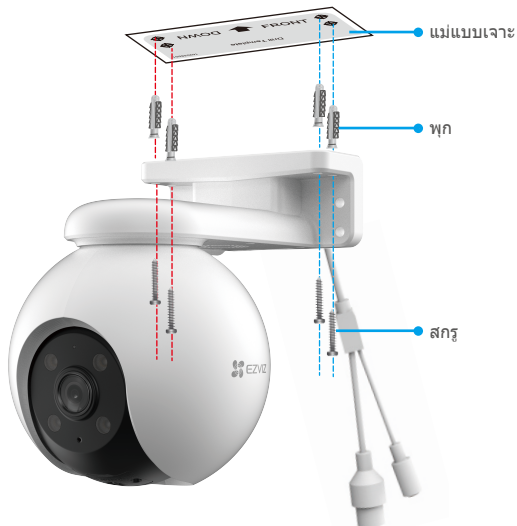
รูปที่ 1 การติดตั้งบนเพดาน
