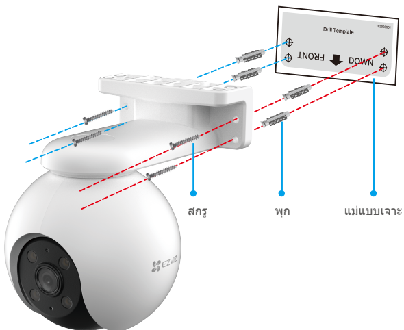
รูปที่ 2 การติดตั้งบนผนัง
